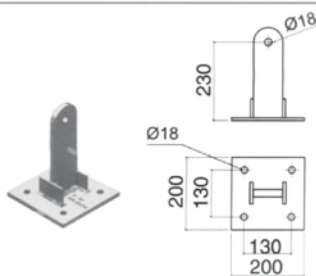
Piastra antipendolo con base piana
