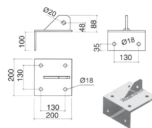
Piastra terminale ad angolo
