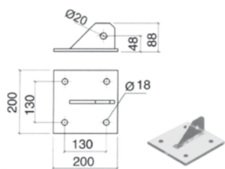
Piastra terminale semplice
