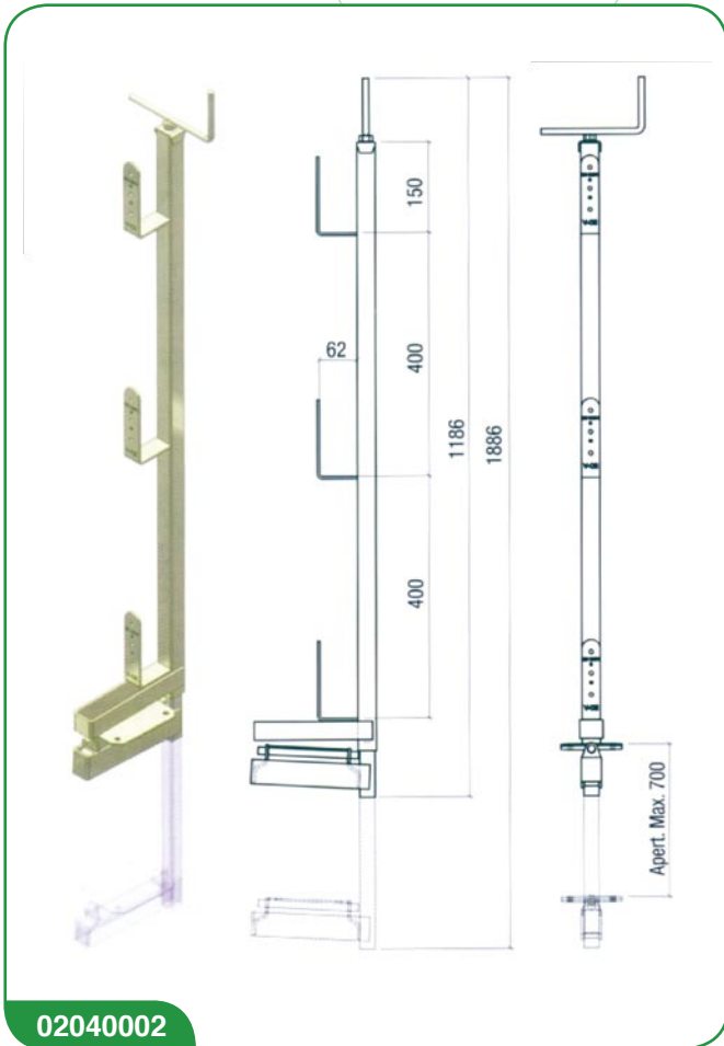
■ Parapetti provvisori zincati H 1,20 mt certificati
