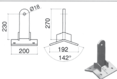
Piastra antipendolo con base doppia incl.
