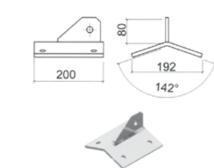
Piastra terminale semplice a doppia falda
