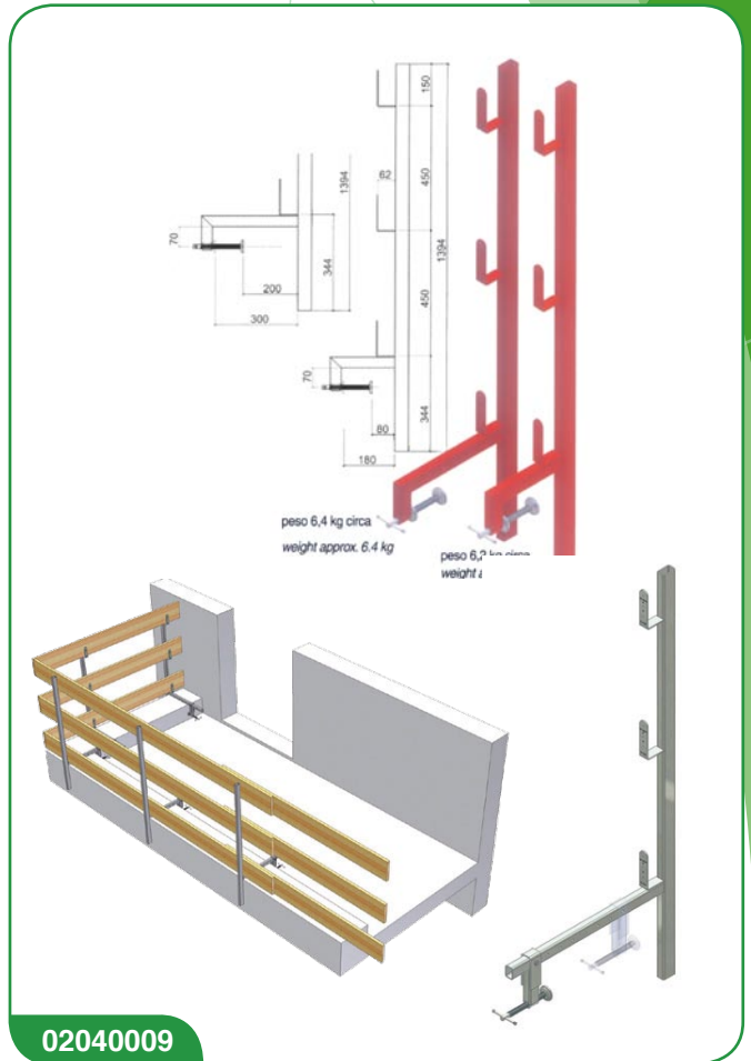
■ Parapetti provvisori per cordoli certificati (ancoraggio da 80 a 180mm. / da 200 a 300mm. / da 80 a 450mm.)
